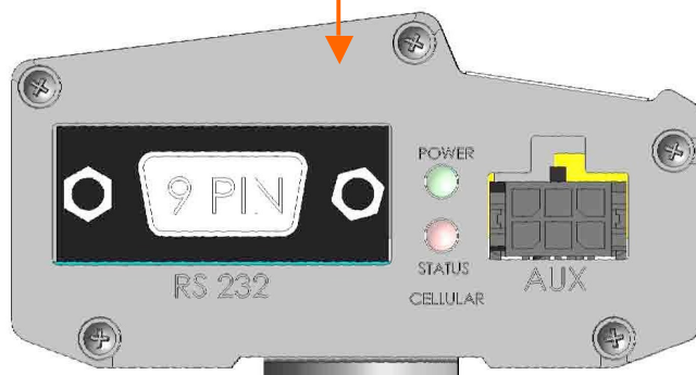
Pinbelegung RS-232 D-Typ 9-pin female RS232
