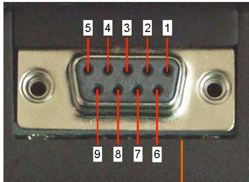
Pinbelegung RS-232 D-Typ 9-pin female RS232
